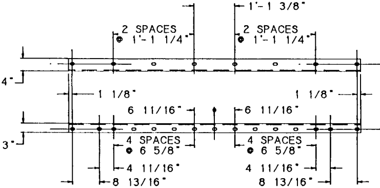
8' STRAIGHT RIB - P.C. 32122
