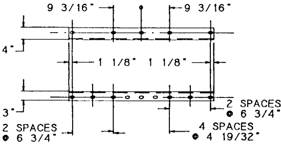
4' STRAIGHT RIB - P.C. 32121
