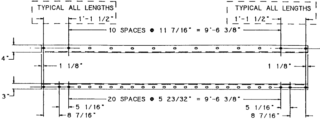
12' STRAIGHT RIB - P.C. 32123
