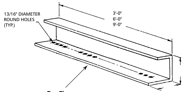
Top Tie
